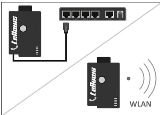
Anschluss mit VoIP (einfache LAN-Verbindung Anrufblocker und Router; Einstellungen am Router für Betrieb notwendig)
